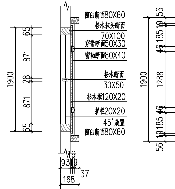
2-2剖面图 1:20
