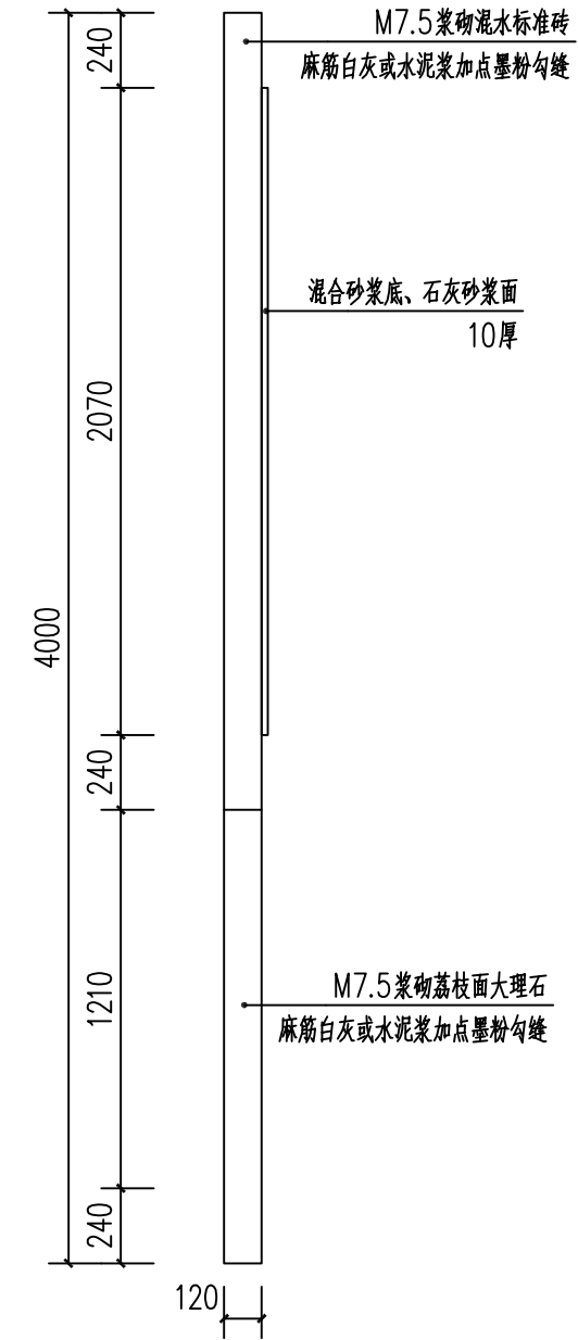
1—1 剖面图 1:25
