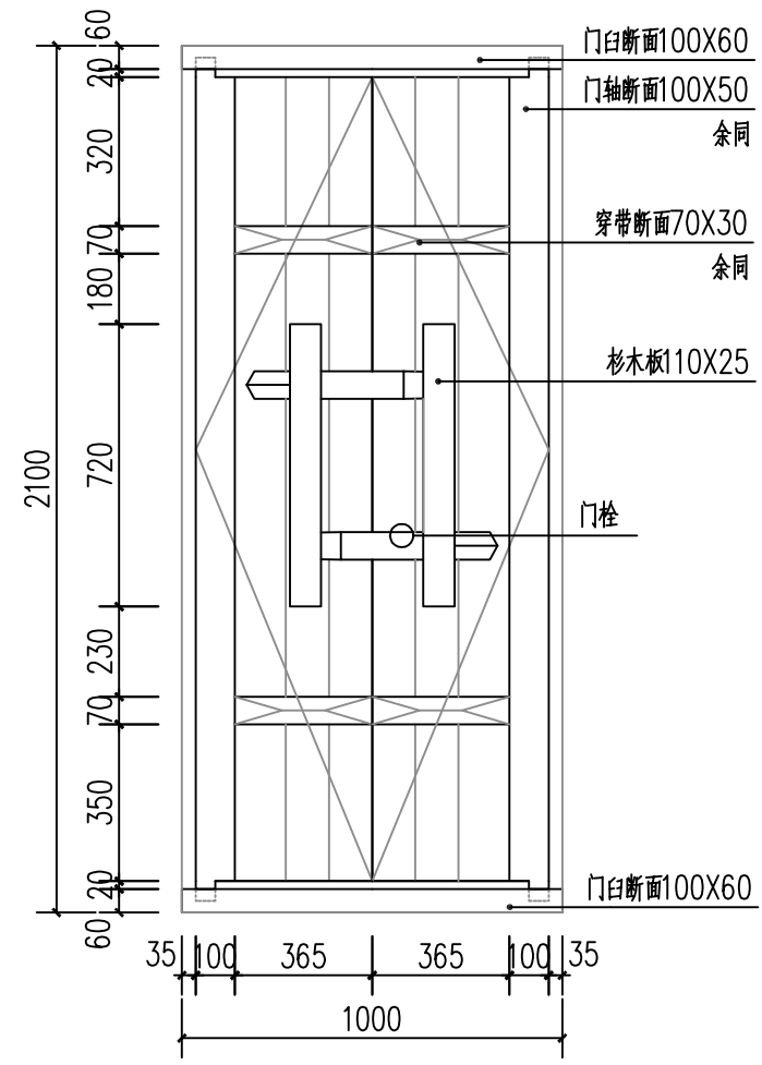
门内立面图 1:20
