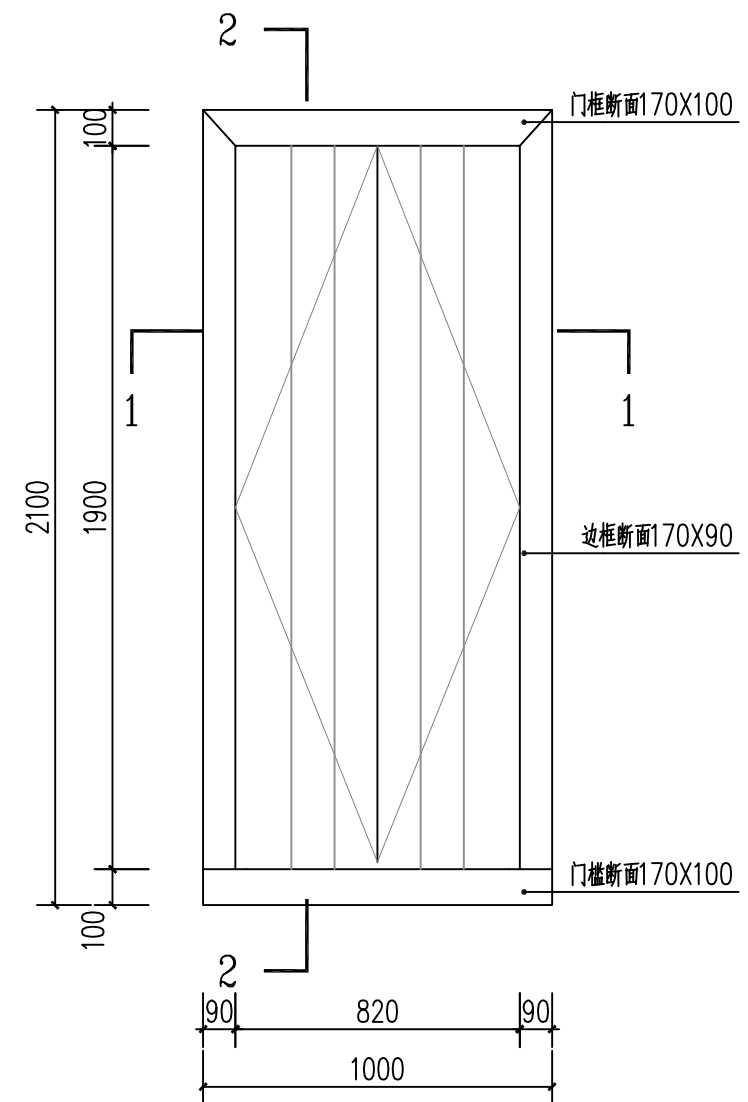
门外立面图 1:20
