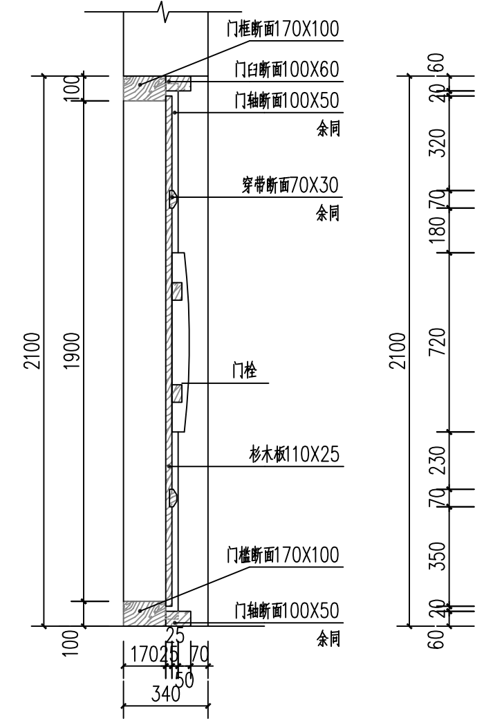
2-2剖面图 1:20
