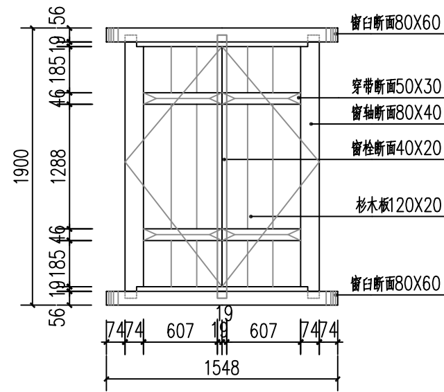
窗内立面图 1:20
