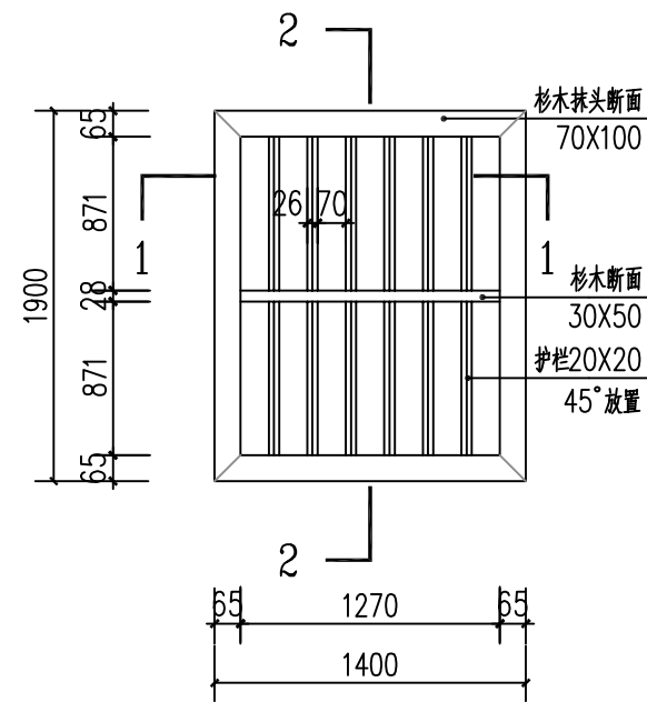
窗外立面图 1:20
