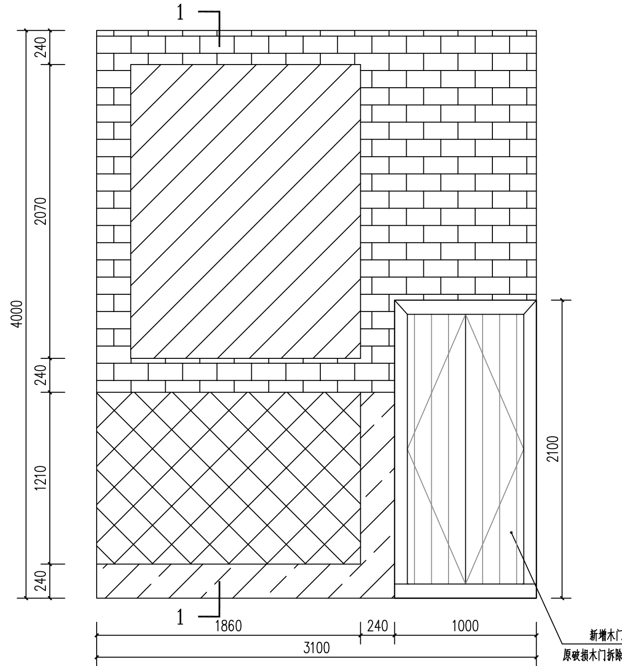
墙面修复立面示意图 1:25
