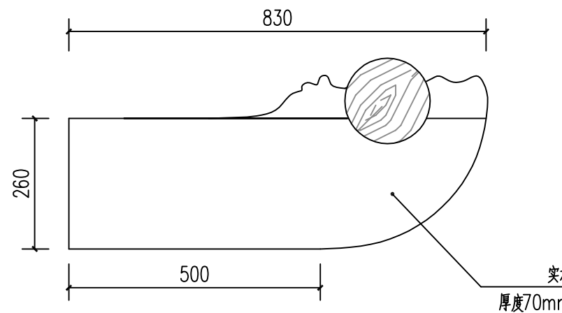
丁头拱大样图 1:10
