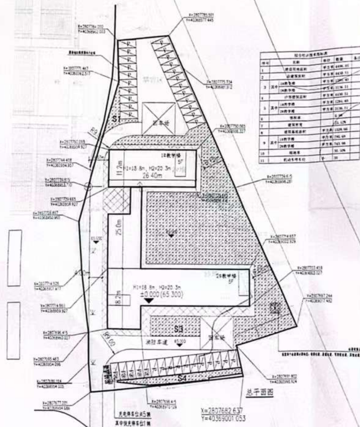
仙游一中1#教学楼、仙游一中2#教学楼总平面图
